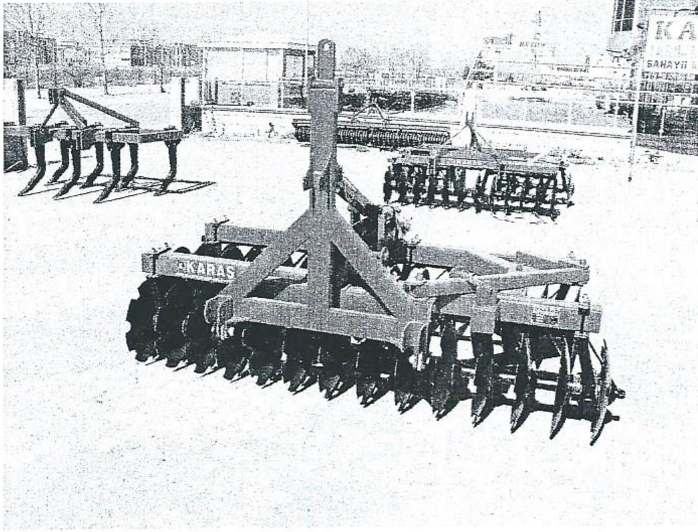
KARAS DİSKARO (28 Diskli, Asılır Tip)
